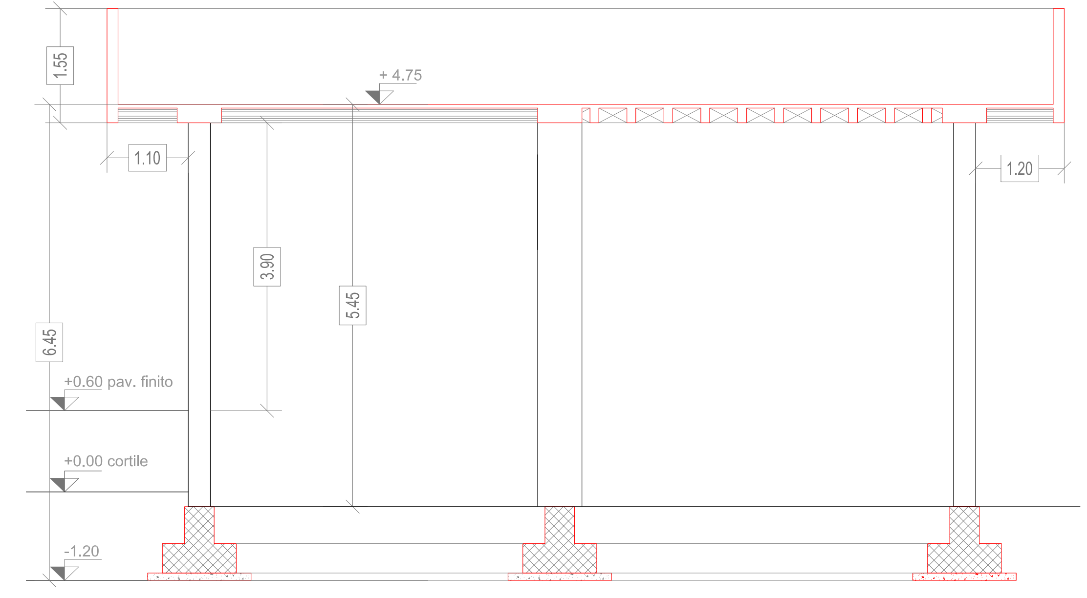
SEZIONE A-A
